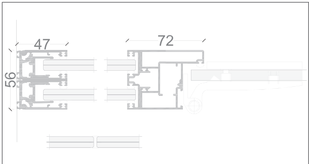
HORIZONTAL SECTION GLASS DOOR
