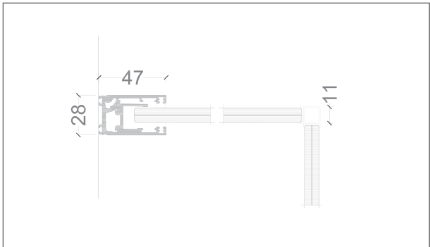
90° ANGLE
